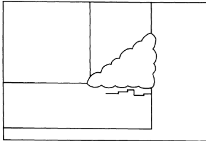
FIG. 5 LAMELLAR TEARING
